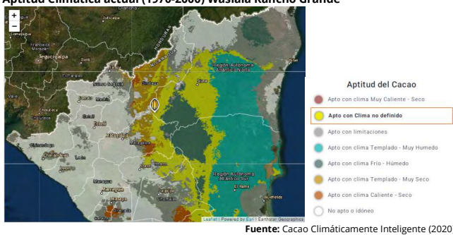
Figura 1 Aptitud Climática actual (1970-2000) Waslala Rancho Grande
